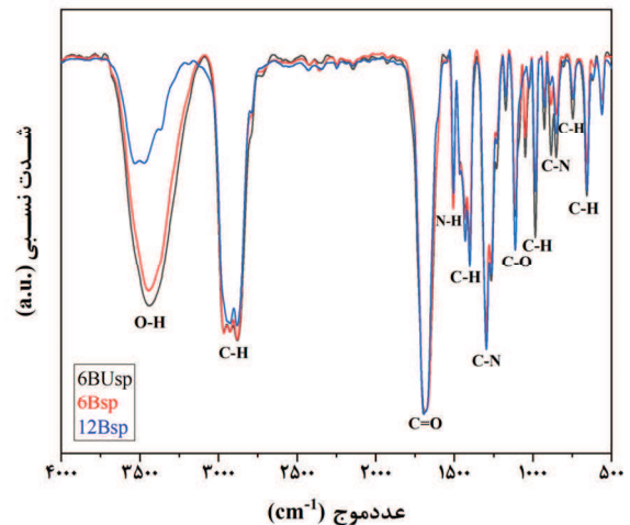
شکل ۴- طیف FTIR نمونه‌های 6BUsp، 6Bsp و 12Bsp
