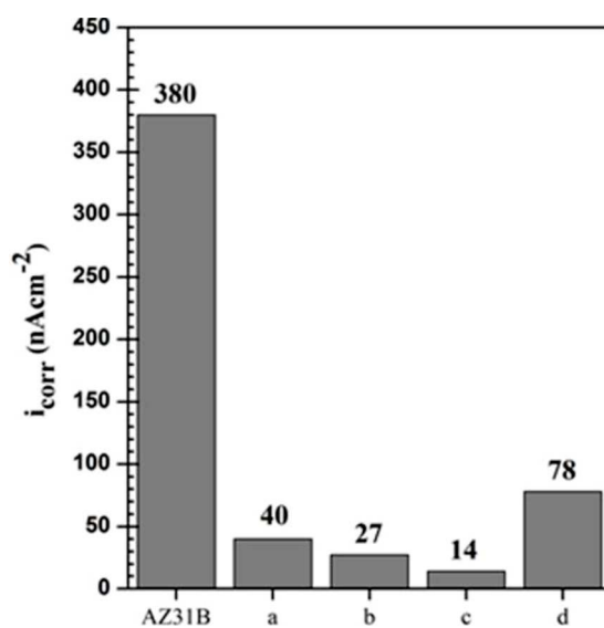
شکل ۸- تغییرات چگالی جریان خوردگی نمونه‌های a-d و AZ31B.
