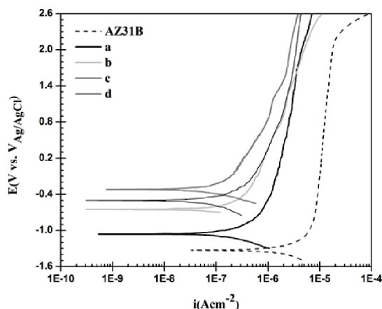
شکل ۷- منحنی‌های پلاریزاسیون پتانسیودینامیک به دست آمده از نمونه‌های a-d و AZ31B در محلول ۰/۰۱ مولار هیدروکسید سدیم در نرخ روبش ۱ میلی‌ولت بر ثانیه.
