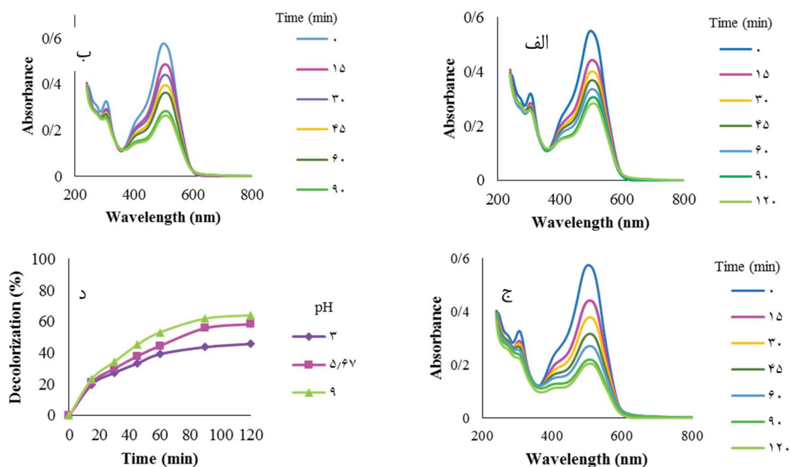
شکل ۶- رنگزدایی رنگزای مستقیم قرمز ۲۳ توسط فوتوکاتالیست سنتز شده به روش هم‌رسوبی با مقادیر مختلف pH (الف) ۳ (ب) ۵/۶۷ (ج) ۹ (د) بررسی اثر مقدار pH بر رنگزدایی
