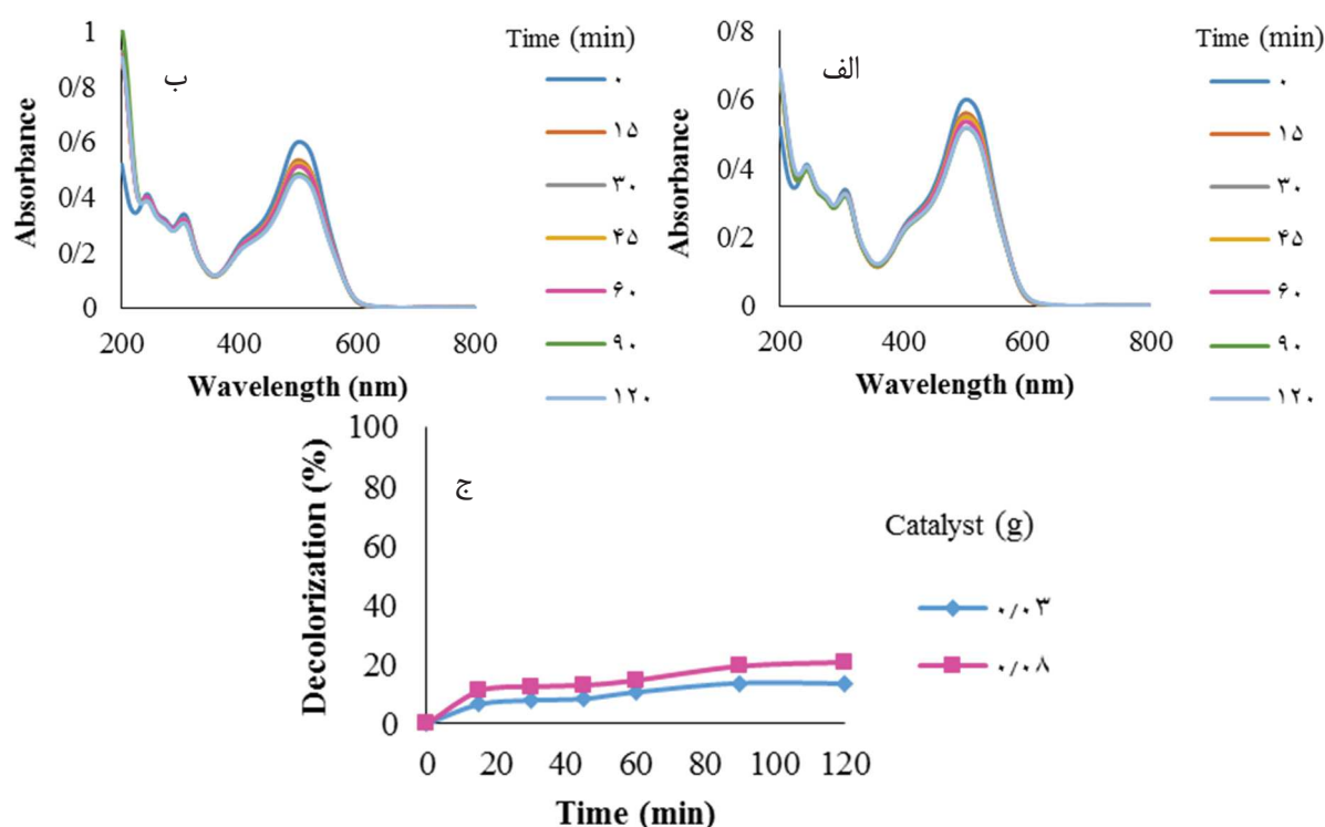
شکل ۸- رنگزدایی رنگزای مستقیم قرمز ۲۳ توسط فوتوکاتالیست سنتز شده به روش هیدروترمال با مقادیر مختلف فوتوکاتالیست (الف) 0.03 \text{ g} (ب) 0.08 \text{ g} (ج) بررسی اثر مقدار فوتوکاتالیست بر رنگزدایی
