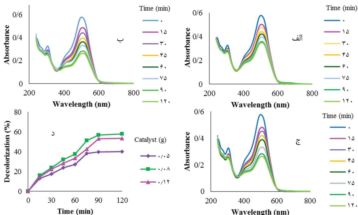
شکل ۵- رنگزدایی رنگزای مستقیم قرمز ۲۳ توسط فوتوکاتالیست سنتز شده به روش هم‌رسوبی با مقادیر مختلف فوتوکاتالیست (الف) ۰/۰۵g (ب) ۰/۰۸g (ج) ۰/۱۲g (د) بررسی اثر مقدار فوتوکاتالیست بر رنگزدایی
