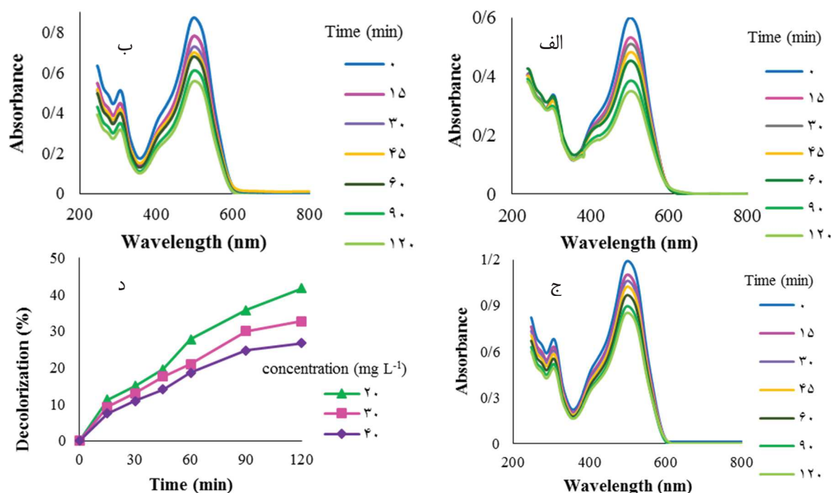
شکل ۱۰- رنگزدایی غلظت‌های مختلف رنگزای مستقیم قرمز ۲۳ توسط فوتوکاتالیست سنتز شده به روش هیدروترمال (الف) 20 \text{ mg L}^{-1} (ب) 30 \text{ mg L}^{-1} (ج) 40 \text{ mg L}^{-1} (د) بررسی اثر میزان غلظت بر رنگزدایی
