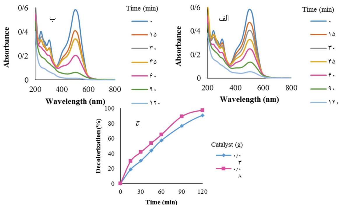
شکل ۱۱- رنگزدایی رنگزای مستقیم قرمز ۲۳ توسط فوتوکاتالیست سنتز شده به روش احتراقی با مقادیر مختلف فوتوکاتالیست (الف) (ب) ۰/۰۳g (ج) بررسی اثر مقدار فوتوکاتالیست بر رنگزدایی
