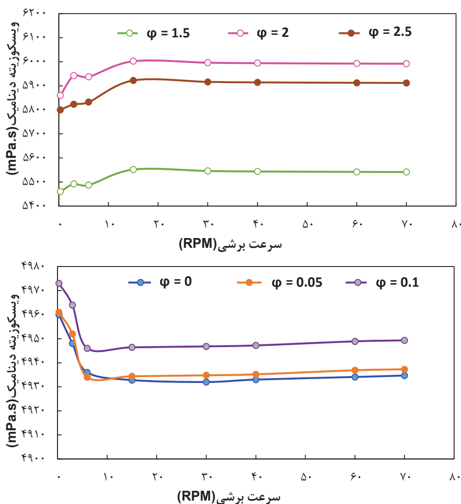
شکل ۶- تغییرات ویسکوزیته نانوسیال به ازای تغییرات نرخ برش و درصد حجمی جامد در دمای ۲۹۸ کلون
