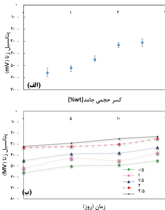
شکل ۴- پتانسیل زتای نانوسیالات هیبریدی بر حسب (الف) کسر حجمی جامد و (ب) زمان.
