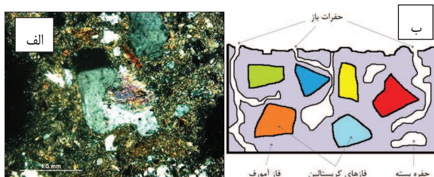
شکل ۱- (الف) بافت زمینه، حفرت (قسمت‌های سیاه رنگ) و فازهای بلورین در تصویر مقطع نازک نمونه سفال تاریخی (میکروسکوپ پلاریزان، آنالیزاتور + پلاریزاتور). (ب) طرح ترسیمی از تخلخل باز و بسته و همچنین فاز آمورف (بافت زمینه) و فاز کریستالین (دانه‌ها) در بافت یک ماده متخلخل مانند سرامیک رسی از منظر میکروسکوپی.
