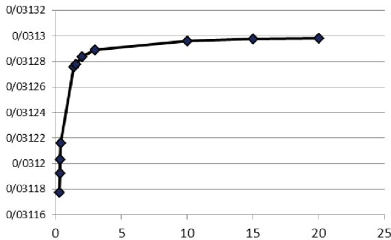
شکل ۱۰- نمودار تابع فشار بخار (atm) درون حفره (محور Y) نسبت به شعاع انحناى مایع (μm) (در اینجا شعاع حفره) (محور X) با افزایش اندازه شعاع.
