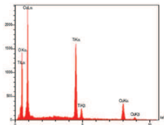
شکل ۹- نمودار EDS فوم مسی آندایز شده توسط جریان مستقیم با پوشش \text{TiO}_2
