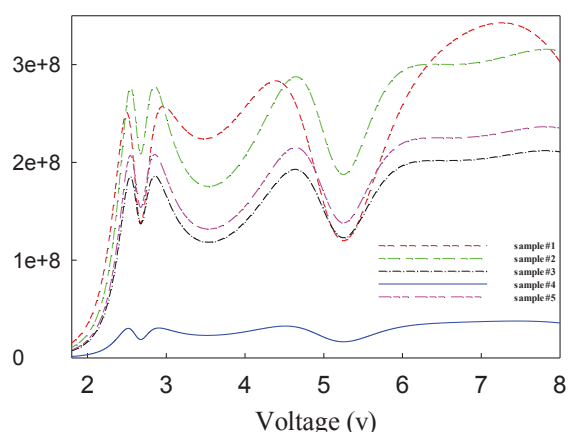
شکل ۸- چگالی جریان نمونه‌های کاشت شده بر حسب ولتاژ اعمالی.
