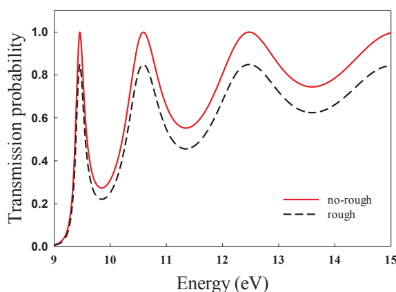
شکل ۵- تاثیر ناهمواری بر احتمال عبور نمونه کاشت نشده.
