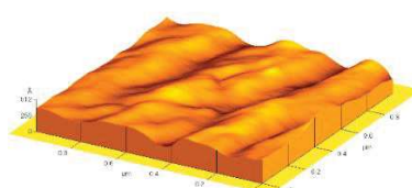
کاشت شده با جریان یونی 5 \times 10^{17}
