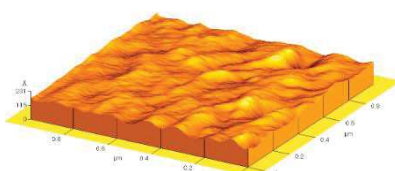
کاشت شده با جریان یونی 3 \times 10^{17}
