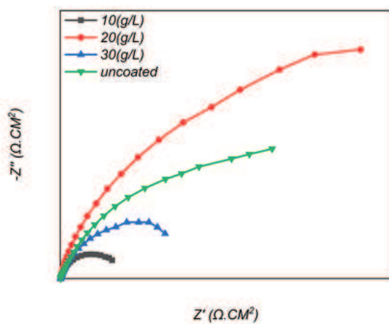
شکل ۳- نمودار نایکویست فولاد بدون پوشش و پوشش کامپوزیتی Ni-P-W-TiO_2 در مقادیر متفاوت اکسید تیتانیوم
