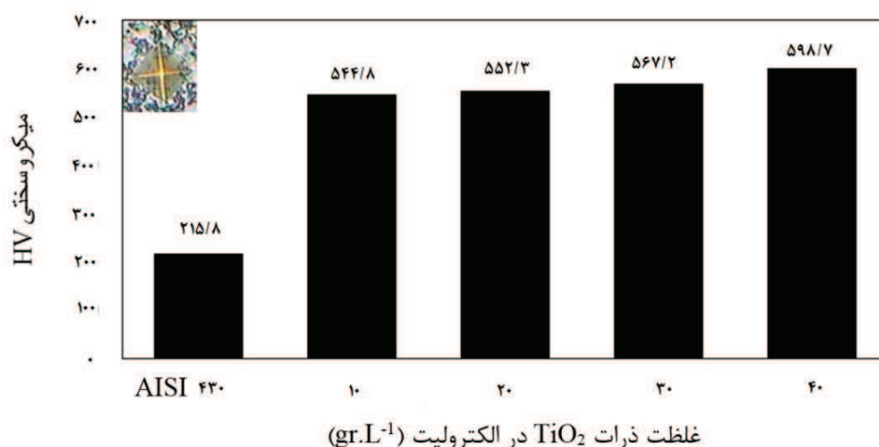
شکل ۶- تاثیر غلظت ذرات \text{TiO}_2 در الکترولیت بر میکروسختی پوشش کامپوزیتی
