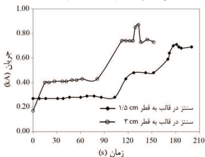
شکل ۳- نمودار جریان در برابر زمان برای نمونه‌های آسیا شده به مدت ۹ ساعت و سپس سنتز شده در دستگاه جرقه پلاسما با قالب به قطر 1/5 و 3 cm، به منظور سنتز درجای کامپوزیت کاربید بور-کاربید سیلیسیم به روش سنتز احتراقی حجمی.
