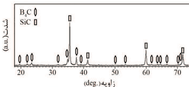
شکل ۴- الگوی XRD پس از اسید شویی نمونه آسیا شده (به مدت ۹ ساعت) و سپس سنتز شده در دستگاه جرقه پلاسما با قالب به قطر 3 cm، به منظور سنتز درجای کامپوزیت کاربید بور-کاربید سیلیسیم به روش سنتز احتراقی حجمی.
