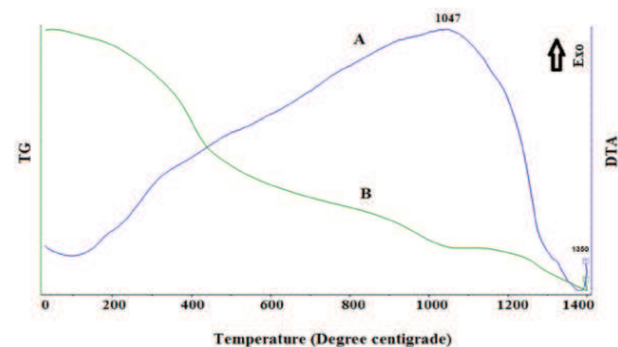
شکل ۶- منحنی‌های آنالیز حرارتی افتراقی و تغییرات وزنی نمونه در دماهای مختلف مربوط به ژل نهایی
