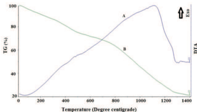
شکل ۶- منحنی‌های آنالیز حرارتی افتراقی و تغییرات وزنی نمونه در دماهای مختلف مربوط به ژل نهایی در شرایط pH=۵
