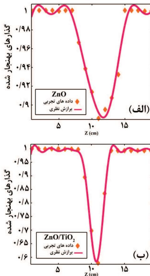
شکل ۷- گذارهای بهنجار شده تجربی روبش Z -دریچه باز به همراه برازش‌های نظری در حضور (الف) نانو ذرات ZnO و (ب) نانو کامپوزیت‌های هسته/پوسته ZnO/TiO 2 .
