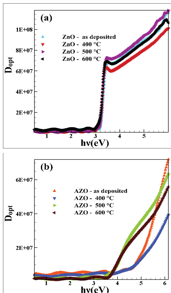
شکل ۱- نمودار چگالی ایتیکی بر حسب انرژی برای لایه های بازپخت شده اکسید روی و اکسید روی تزریق شده با آلومینیوم در دمای اتاق، ۴۰۰، ۵۰۰ و ۶۰۰ درجه سانتی گراد.
