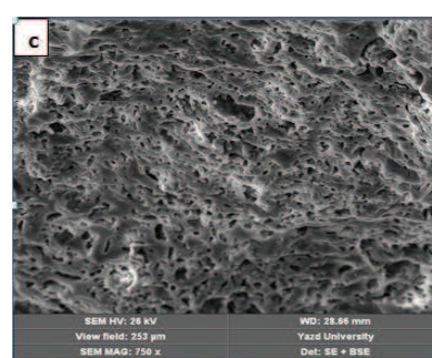
شکل ۵- تصویر SEM سه نمونه ۱۴ (a) و ۱۶ (b) و ۱۷ (c) در دمای 1186^\circ\text{C} در بزرگ‌نمایی 750\times .
