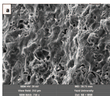
شکل ۵- تصویر SEM سه نمونه ۱۴ (a) و ۱۶ (b) و ۱۷ (c) در دمای 1186^\circ\text{C} در بزرگ‌نمایی 750\times .
