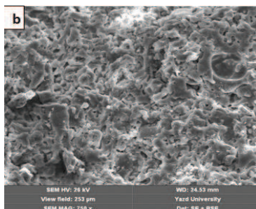
شکل ۶- تصویر SEM سه نمونه ۱۴ (a) و ۱۶ (b) و ۱۷ (c) در دمای 1137^\circ\text{C} در بزرگ‌نمایی 750\times .
