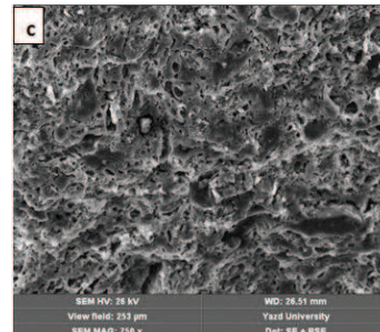
شکل ۶- تصویر SEM سه نمونه ۱۴ (a) و ۱۶ (b) و ۱۷ (c) در دمای 1137^\circ\text{C} در بزرگ‌نمایی 750\times .
