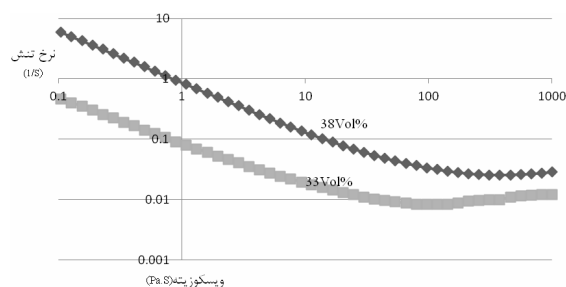
شکل ۳- تغییرات گرانیروی بر حسب نرخ تنش در بارهای جامد ۳۸ vol% و ۳۳ vol%
