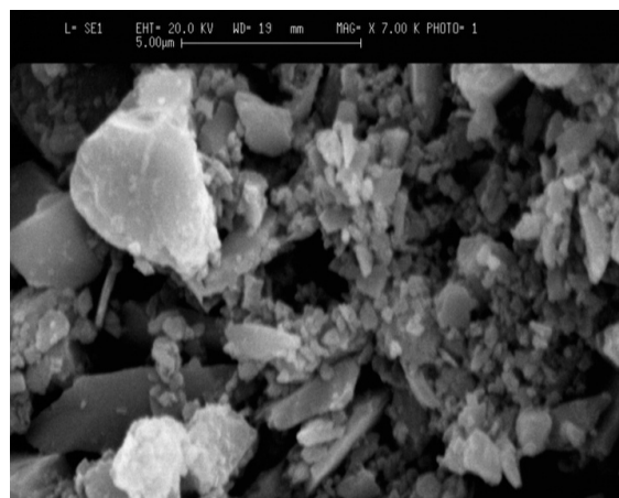
شکل ۸- ریزساختار نمونه ریخته‌گری ژلی شده با بار
