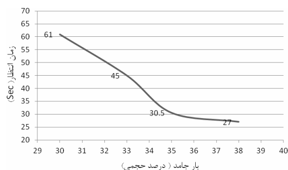
شکل ۴- زمان انتظار دوغاب‌های سیلیسیم
