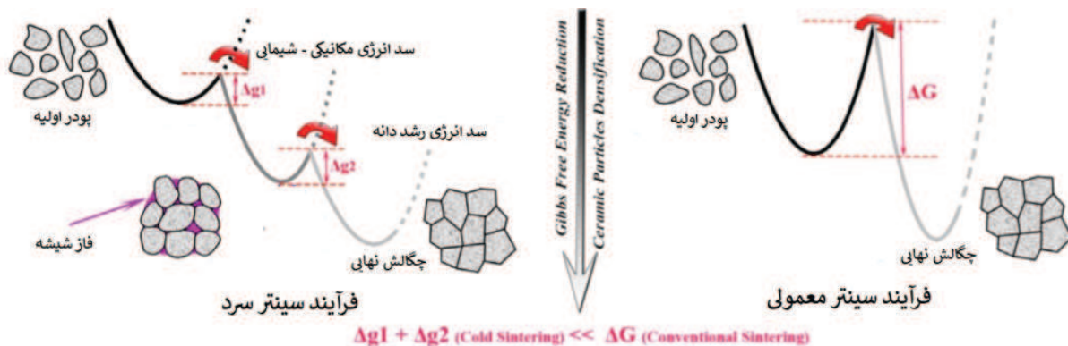
شکل ۴- تغییرات انرژی آزاد گیبس در طول فرآیند سینتر سرد [۳۲].
