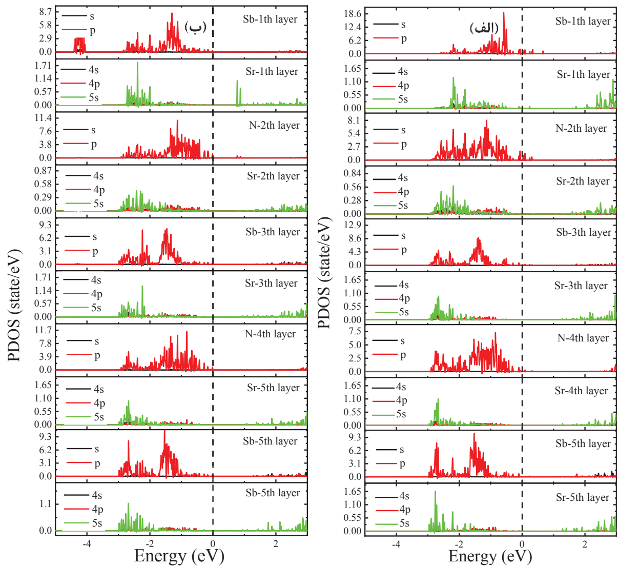
شکل ۴- چگالی حالت‌های جزئی الکترونی ۵ لایه بالایی سطح (الف) خنثی نشده و (ب) خنثی شده توسط اتم‌های هیدروژن با پایانه
