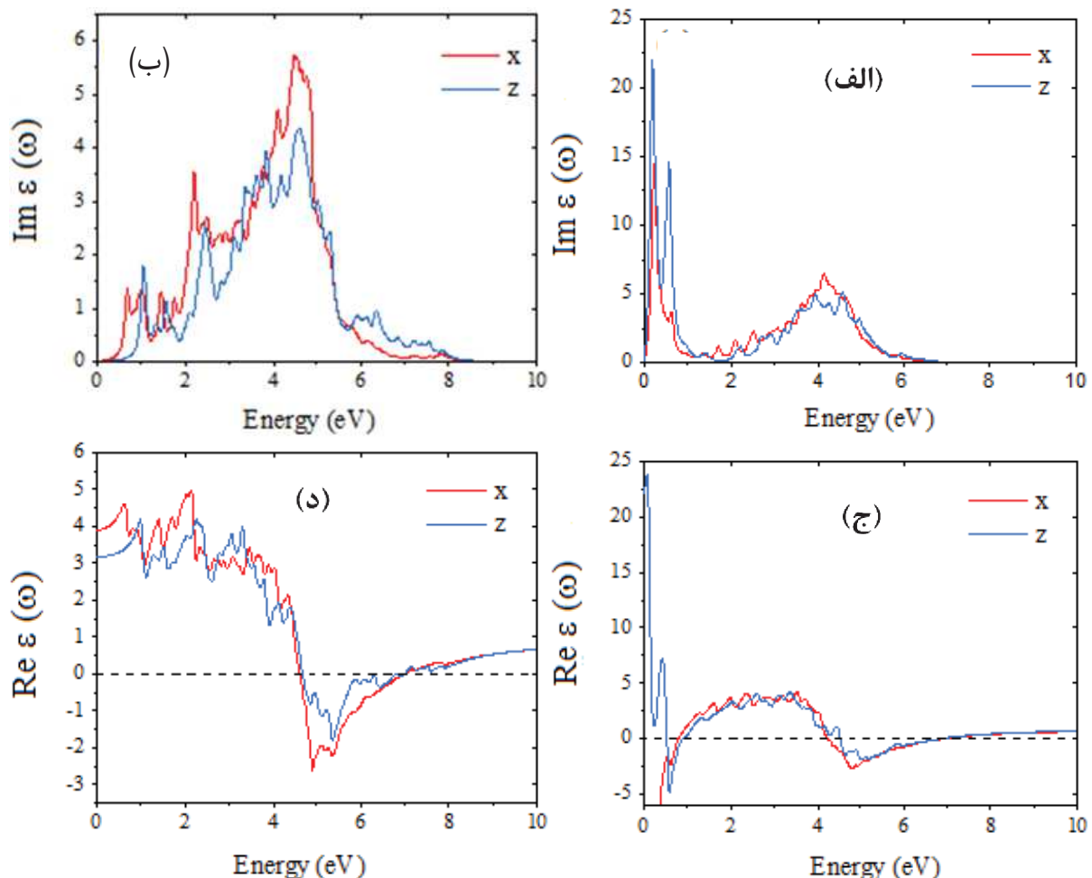
شکل ۶- الف) بخش موهمی تابع دی‌الکتریک سطح خنثی نشده، (ب) خنثی شده، (ج) بخش حقیقی تابع دی‌الکتریک سطح خنثی نشده، و (د) خنثی شده با پایانه SbSr
