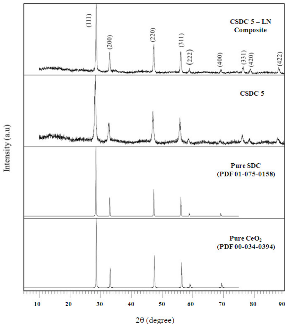
شکل ۱- الگوهای XRD نمونه‌های CSDC 5 و CSDC 5-LN به همراه الگوی مرجع
