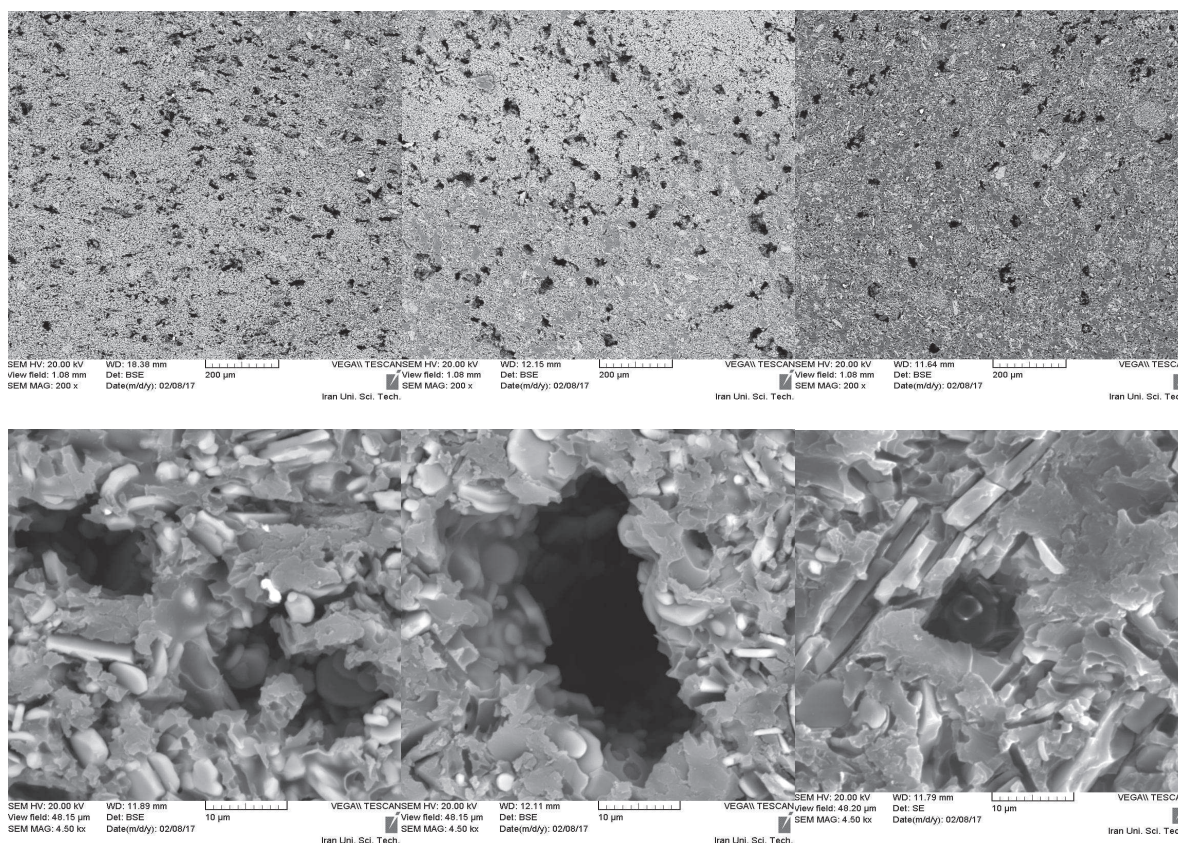
شکل ۴- تصاویر SEM - نمونه‌های (الف) A، (ب) B، (پ) C زینتر شده در دمای 1500^{\circ}\text{C} (تصاویر نمونه‌ها از سطح مانت شده و در دو بزرگنمایی 200\times و 450\times گرفته شده است).
