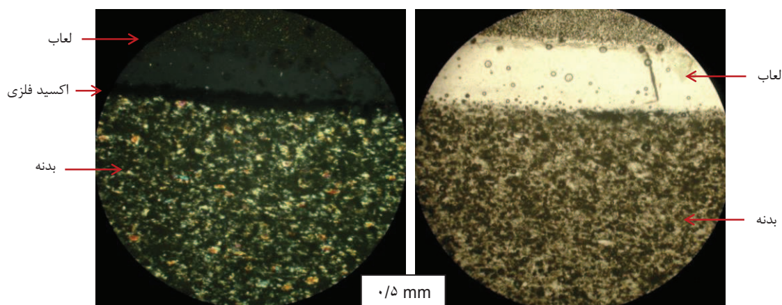
شکل ۱۲ - چپ: فتومیکروگراف نمونه شماره ۲، نور XPL، طول میدان دید ۲/۷ mm، بافت سیلتی و همگن، قطعات فراوان کوارتز ریزدانه و تک بلور در خمیره سفال. در حاشیه بالایی نمونه لایه لعاب شیشه‌ای همراه با یک لایه اکسید فلزی تیره رنگ در حد فاصل بین بدنه و لعاب. راست: فتومیکروگراف نمونه شماره ۲، نور PPL، طول میدان دید ۲/۷ mm، لعاب شیشه‌ای به رنگ روشن.
