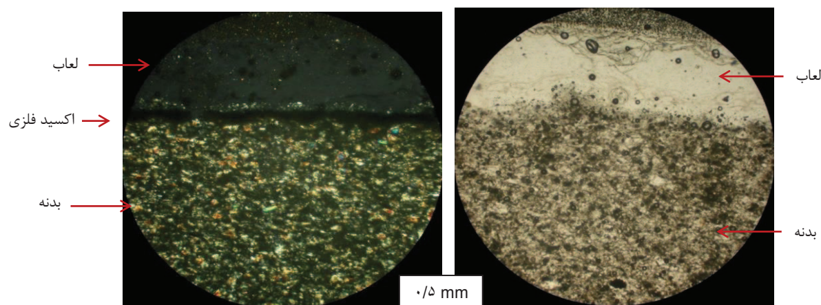
شکل ۱۱ - چپ: فتومیکروگراف نمونه شماره ۱، نور XPL، طول میدان دید ۲/۷ mm، بافت سیلتی و همگن، قطعات فراوان کوارتز ریزدانه و تک بلور در خمیره سفال. در حاشیه بالایی نمونه لایه لعاب شیشه‌ای همراه با یک لایه اکسید فلزی تیره رنگ در حد فاصل بین بدنه و لعاب. راست: فتومیکروگراف نمونه شماره ۱، نور PPL، طول میدان دید ۲/۷ mm، تصویر میکروسکوپی در نور پلاریزه، لعاب شیشه‌ای به رنگ روشن.
