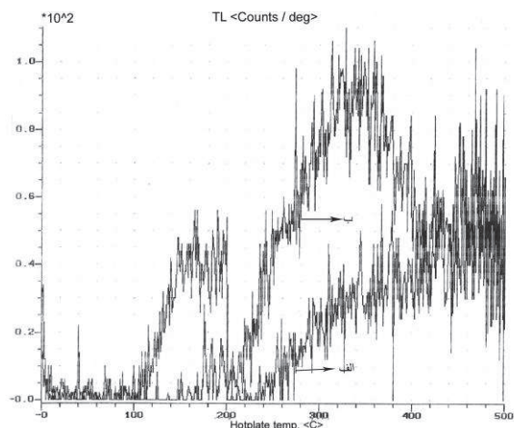
شکل ۵- نمودار ترمولومینسانس نمونه شماره ۲ (نگارندگان)
