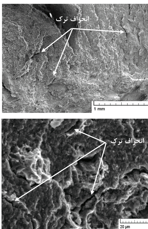
شکل ۱۵- تصویر سطح شکست نمونه‌ی Al_{50}B_4C_{50} در دو بزرگنمایی مختلف.
