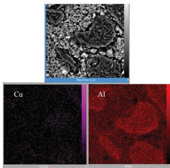
شکل ۹- تصویر میکروسکوپ الکترونی روبشی از نمونه‌ی \text{Al5083-5\%B}_4\text{C-50\%Al2024} و نقشه عنصری این نمونه و حضور
