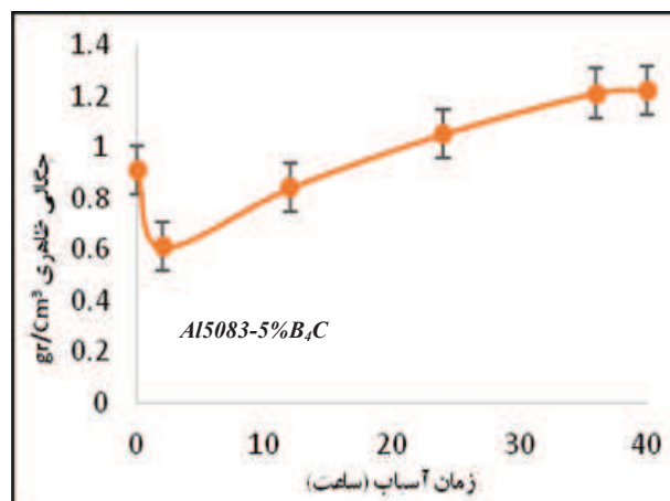
شکل ۵- نمودار وضعیت چگالی ظاهری پودر کامپوزیتی Al_{50}B_{48}C_{2} پس از ۳۶ ساعت آسیاب مکانیکی
