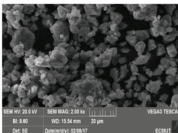
شکل ۲- مورفولوژی نمونه‌ی Al_{50}B_{43}C_7 پس از ۳۶ ساعت آسیاب مکانیکی.
