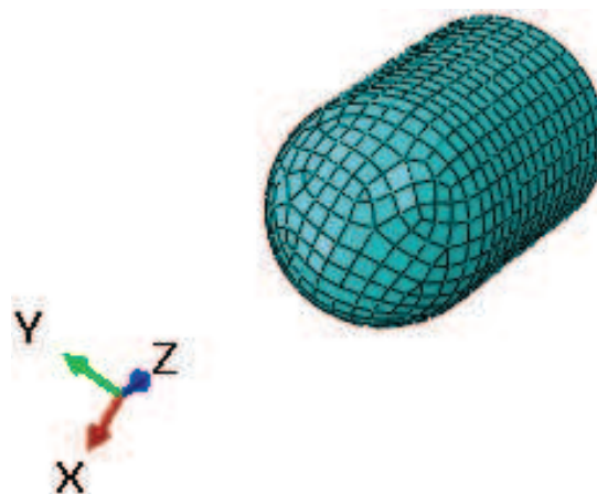
شکل ۱- مش‌بندی پرتابه
