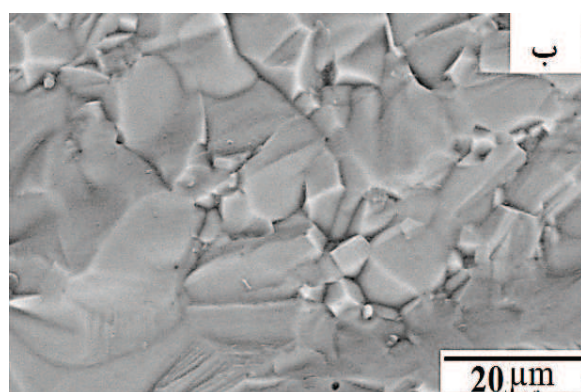
شکل ۲- تصاویر SEM از سطح شکست قطعه یگ شفاف، الف) قبل از آنیل ب) بعد از فرآیند آنی
