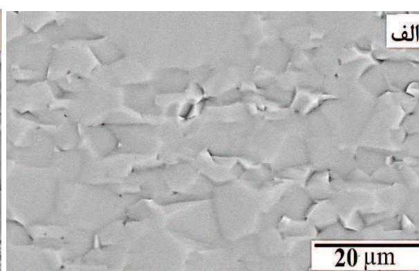
شکل ۲- تصاویر SEM از سطح شکست قطعه یگ شفاف، الف) قبل از آنیل ب) بعد از فرآیند آنی
