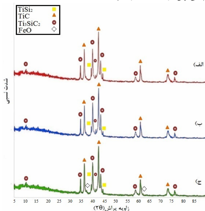
شکل ۳- الگوهای XRD برای نمونه‌های عملیات حرارتی شده در دمای 1100^\circ\text{C} به مدت یک ساعت از نمونه‌های پودری آسیاکاری شده در مدت زمان‌های الف) ۳۰ ساعت، ب) ۴۰ ساعت و ج) ۵۰ ساعت.
