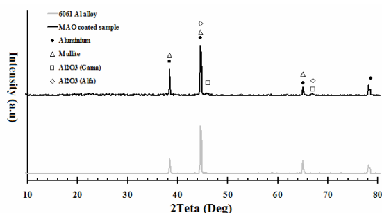
شکل ۱- الگوی پراش اشعه ایکس زیرلایه و پوشش ایجاد شده به روش میکرو قوس الکتریکی روی آلیاژ آلومینیوم ۶۰۶۱
