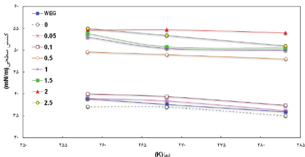
شکل ۸- کشش سطحی سیال پایه بدون سورفکتانت (WEG)، سیال پایه حاوی سورفکتانت ( \phi=0 ) و نانوسیالات هیبریدی با کسرهای مختلف حجمی جامد به صورت تابعی از دما.
