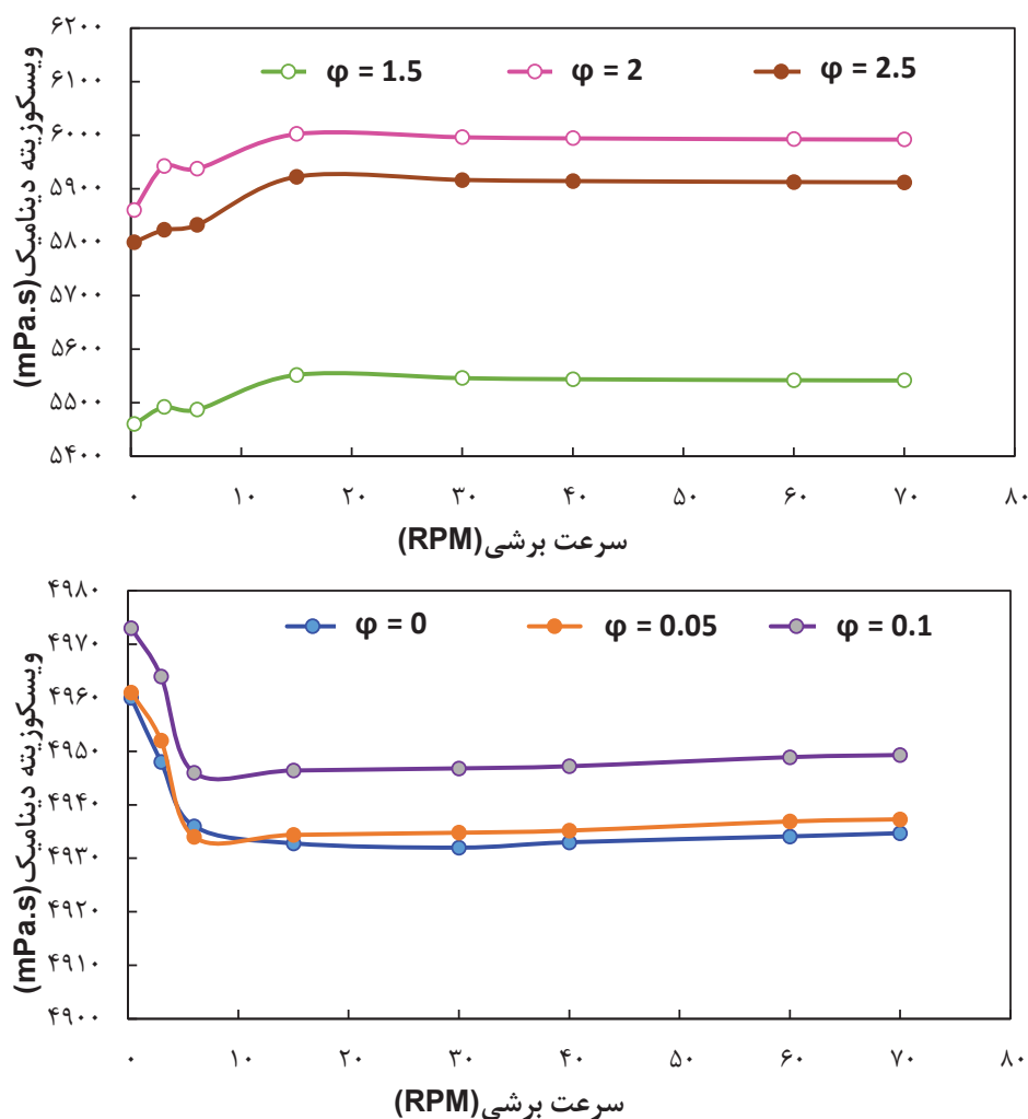
شکل ۶- تغییرات ویسکوزیته نانوسیال به ازای تغییرات نرخ برش و درصد حجمی جامد در دمای ۲۹۸ کلوین
