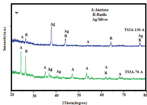
شکل ۱- الگوی پراش پرتو ایکس (الف) نانو کامپوزیت \text{TiO}_2\text{-SiO}_2\text{-5\%Ag} (ب) نانو کامپوزیت \text{SiO}_2\text{-TiO}_2
