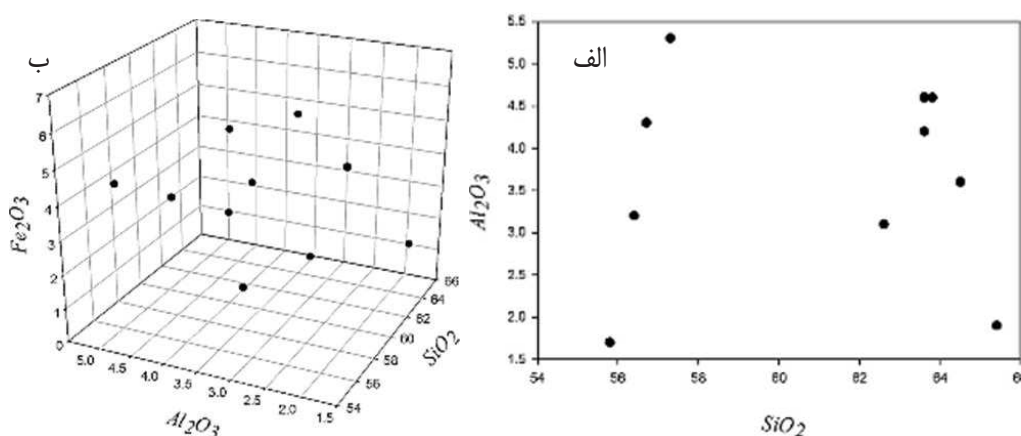
شکل ۲- نمودار پراکندگی نسبت SiO_2 - Al_2O_3 (الف) و SiO_2 - Al_2O_3 - Fe_2O_3 (ب) در نمونه‌های مورد مطالعه برحسب درصد وزنی (Wt%).
