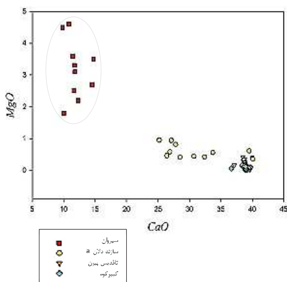
شکل ۴- موقعیت قرارگیری نمونه‌های شیشه سیروان نسبت به نمونه سنگ‌های کربناته کبیرکوه، تاقدیس پیون و چاه دانان - a در سازند ایلام [۳۰] بر اساس درصد وزنی (Wt%) در نمودار CaO- MgO.
