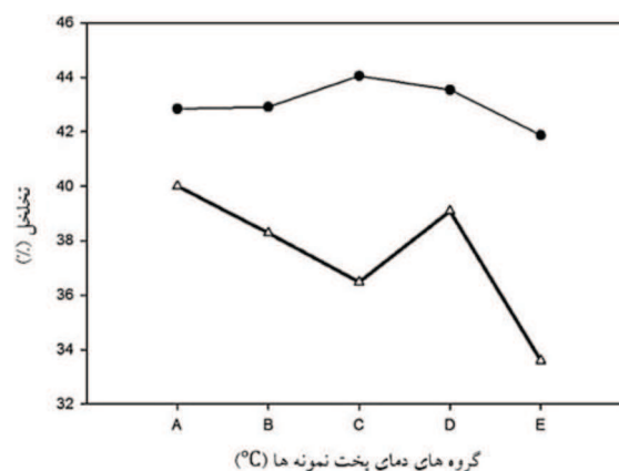
شکل ۲- نمودار تغییرات میانگین درصد تخلخل نمونه‌ها با دو روش اندازه‌گیری تخلخل سنجی جیوه (●) و تخلخل سنجی به روش غوطه‌وری (Δ). A: دمای ۸۵۰°C، B: دمای ۹۰۰°C، C: دمای ۹۵۰°C، D: دمای ۱۰۰۰°C، E: ۱۰۵۰°C.
