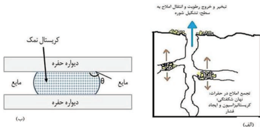
شکل ۷- (الف) طرح ترسیمی از شکل‌گیری شوره در سطح و نهان شکستگی‌ها در حفرات داخلی یک شیء متخلخل از منظر میکروسکوپی و ایجاد تنش ناشی از کریستالیزاسیون به دیواره حفرات. (ب) طرح ترسیمی از کریستال تشکیل شده در یک حفره استوانه‌ای شکل (براساس [۲۰]).
