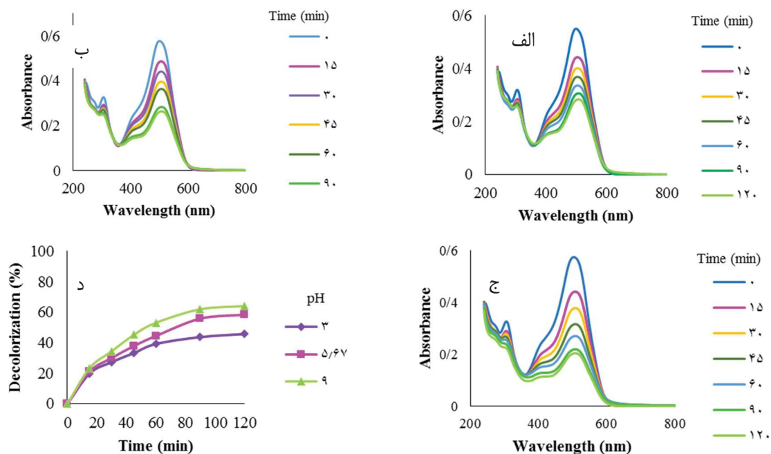
شکل ۶- رنگزدایی رنگزای مستقیم قرمز ۲۳ توسط فوتوکاتالیست سنتز شده به روش هم‌رسوبی با مقادیر مختلف pH (الف) ۳ (ب) ۵/۶۷ (ج) ۹ (د) بررسی اثر مقدار pH بر رنگزدایی
