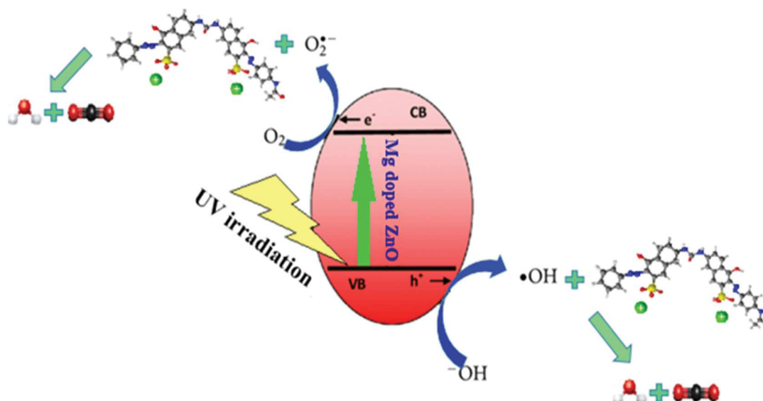
شکل ۱۴- شماتیک بیان کننده مکانیزم رنگدایی رنگزای مستقیم قرمز ۲۳ توسط Mg-ZnO سنتز شده به روش احتراقی
