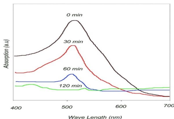
شکل ۸- تصویر طیف‌سنجی نور مرئی و فرابنفش اسید قرمز
