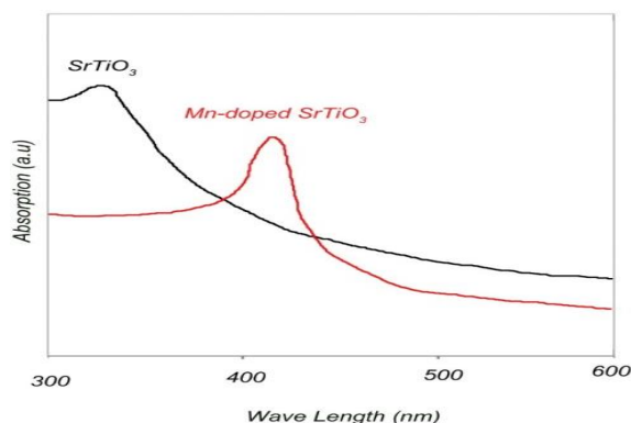
شکل ۹- تصویر طیف‌سنجی نور مرئی و فرابنفش کامپوزیت پروسکایت استرانسیوم تیتانات-منگنز
