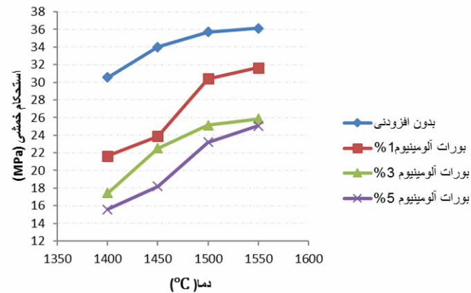
شکل ۳- استحکام خمشی نمونه‌های حاوی افزودنی بورات آلومینیوم در مقایسه با نمونه بدون افزودنی پس از پخت در دماهای مختلف
