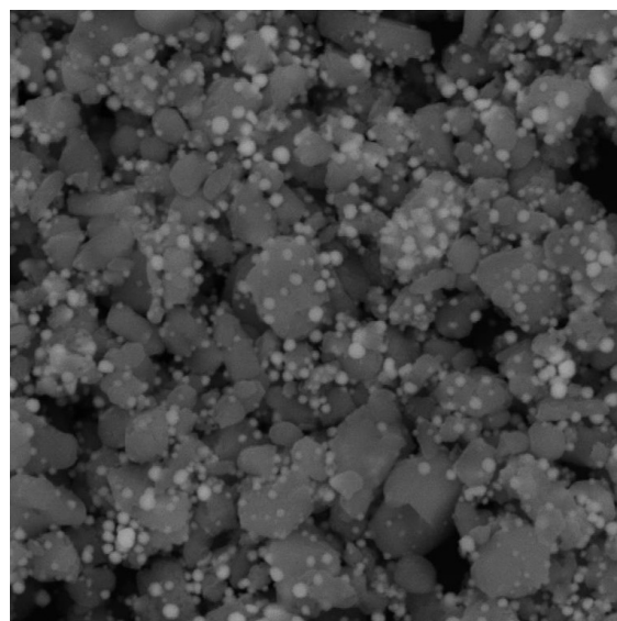
شکل ۸- ریزساختار پودر آلومینا-کبالت احیاء شده از روش احیاء واکنشی و دردمای ۱۱۰۰°C و به مدت ۲ ساعت
