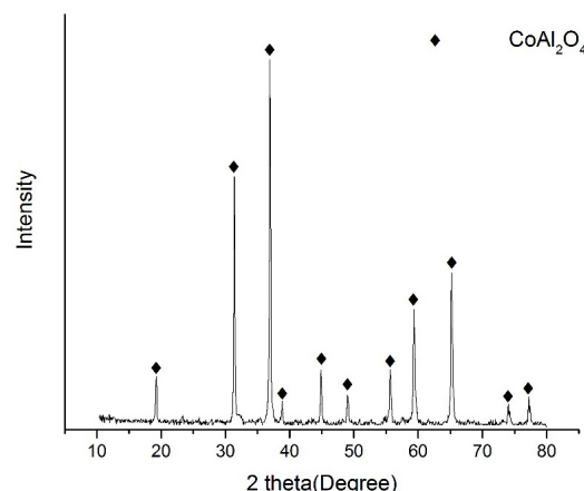
شکل ۱- الگوی پراش اشعه ایکس از اسپینل آلومینات کبالت سنتزی به روش سیتراست سل-ژل کلسینه شده در دمای 700^{\circ}\text{C}
