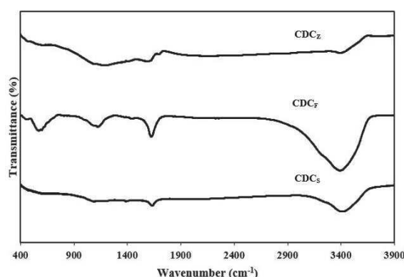
شکل ۴- طیف نمونه‌های FTIR، CDCs، CDCF و CDCz
