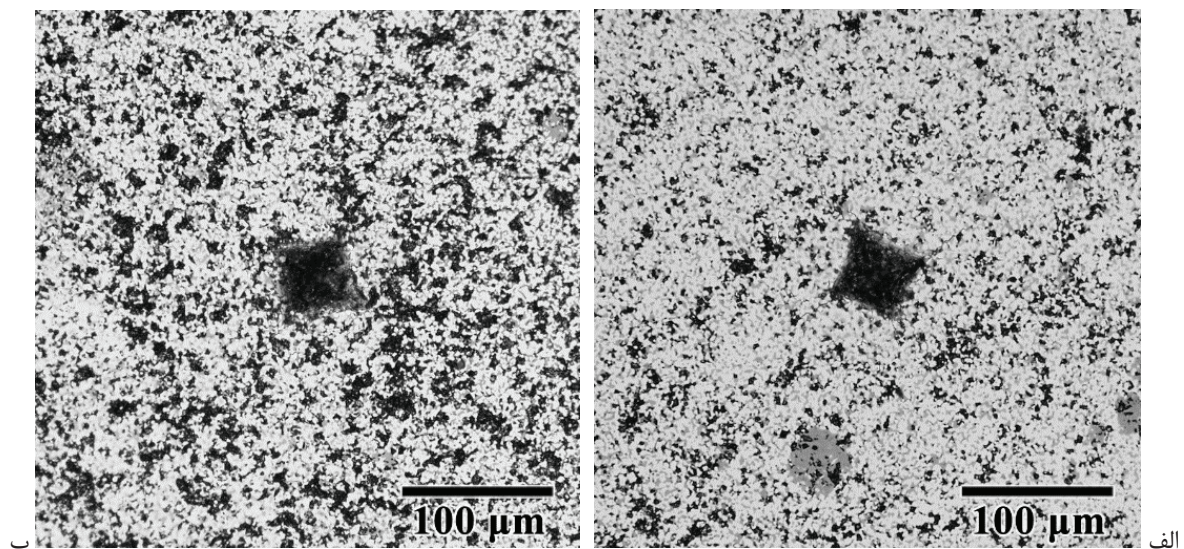
شکل ۳- تصاویر میکروسکوپ نوری از محل اثر فرو رونده ویکرز برای سختی‌سنجی نمونه‌های کامپوزیتی (الف) فاقد افزودنی نانو گرافیت و (ب) دارای 2/5 درصد وزنی افزودنی نانو گرافیت.
