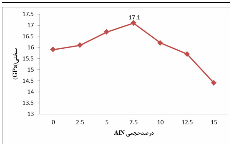
شکل ۱۱- مقادیر سختی بر حسب تغییرات درصد حجمی AlN در دمای زینتر 2150^\circ C درجه سانتیگراد
