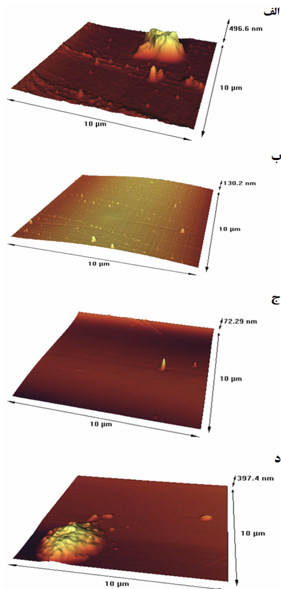
شکل ۳- تصاویر AFM الف) پوشش تیتانیا-آلومینا. ب) پوشش تیتانیا-آلومینا حاوی ۱/۲ درصد بنزوتريازول. ج) پوشش تیتانیا-آلومینا حاوی ۳/۶ بنزوتريازول. د) پوشش تیتانیا-آلومینا حاوی ۴/۸ بنزوتريازول.
