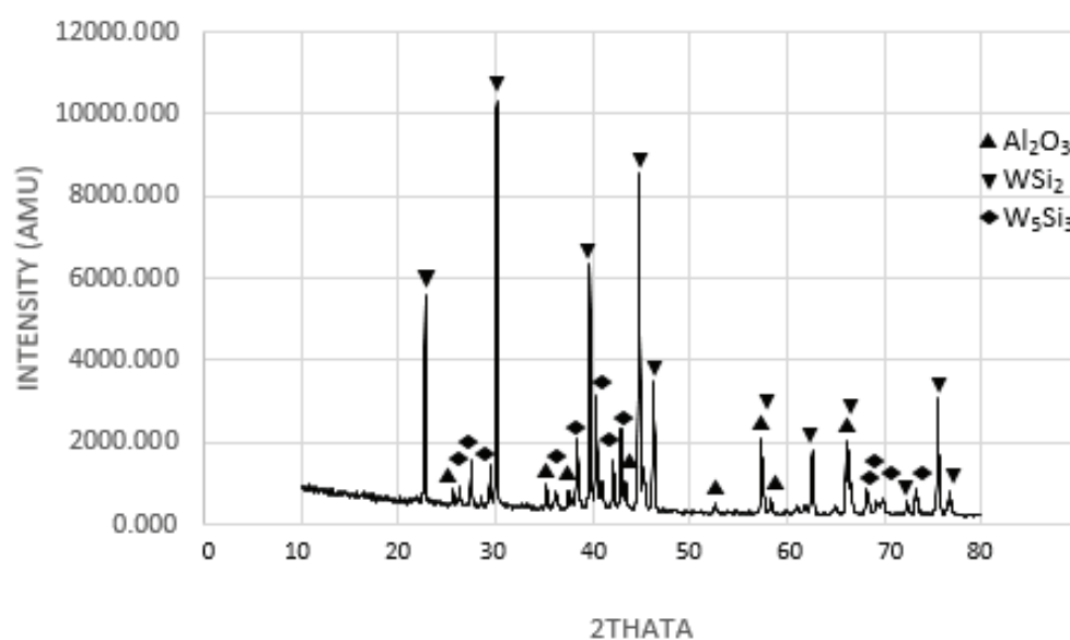
شکل ۲- آنالیز XRD نمونه‌ی DTA و TGA تا دمای 1300^{\circ}\text{C} و سرعت گرمایش 20^{\circ}\text{C. min}^{-1} تحت اتمسفر آرگون در سیستم .ASW
