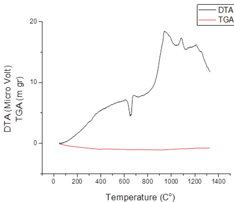
شکل ۱- آنالیزهای DTA و TGA تا دمای 1300^{\circ}\text{C} و سرعت گرمایشی 20^{\circ}\text{C. min}^{-1} تحت اتمسفر آرگون در سیستم .ASW
