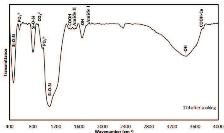
شکل ۱۱- الگوهای FTIR بعد از غوطه‌وری در محلول SBF به مدت ۱۷ روز
