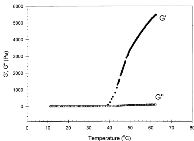
شکل ۱- تغییرات G' و G'' بر حسب دما در محلول کایتوسان/ \beta -GP [۱۵]
