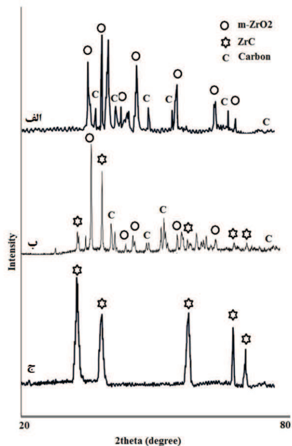
شکل ۷- الگوی XRD نمونه‌های عملیات حرارتی شده در دماهای (الف) 1200^\circ\text{C} ، (ب) 1320^\circ\text{C} و (ج) 1380^\circ\text{C}
