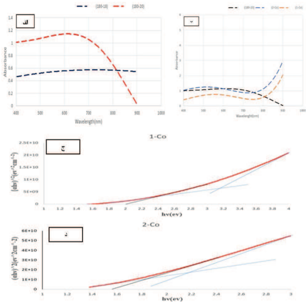
شکل ۵- الف) مقایسه میزان جذب دو نمونه سنتز شده به مدت ۱۸ و ۲۰ ساعت (ب) طیف جذب نمونه های سنتز شده \text{CuIn}_{1-x}\text{Co}_x\text{S}_2 و x=0/2 و مقایسه سه نمونه ۲۰-۱۸۰ و 1-\text{Co} و 1-\text{Co} (ج و د) شکاف انرژی نمونه های سنتز شده \text{CuIn}_{1-x}\text{Co}_x\text{S}_2 (الف) x=0/1 (ب) x=0/2
