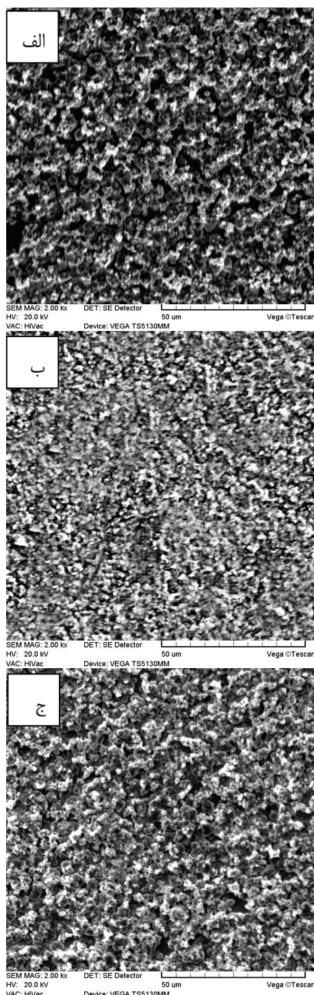
شکل ۱- تصاویر SEM مربوط به مورفولوژی سطح پوشش \text{Ni-P-W-TiO}_2 در غلظت (الف) \text{g/L TiO}_2 = 10 ، (ب) \text{g/L TiO}_2 = 20 و (ج) \text{g/L TiO}_2 = 30
