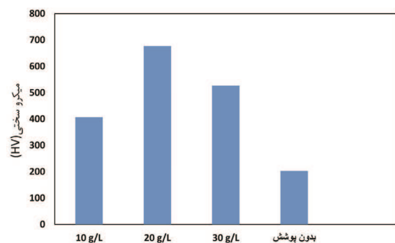
شکل ۶- تغییرات میکروسختی بر حسب غلظت اکسید تیتانیوم موجود در محلول آبکاری برای نمونه‌های بدون پوشش و نمونه‌های پوشش داده شده
