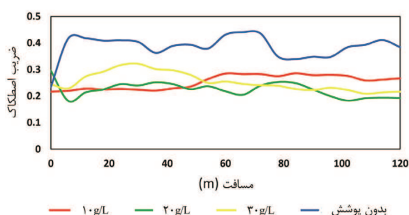
شکل ۸- تغییرات ضریب اصطکاک بر حسب مسافت سایش برای نمونه بدون پوشش و نمونه‌های پوشش داده شده در غلظت‌های ۱۰، ۲۰ و ۳۰ g/L \text{TiO}_2
