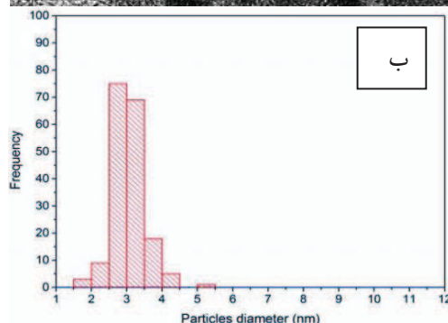
شکل ۲- الف) تصویر TEM از Au_{101}/AC فعال شده (شسته شده با تولوئن و پس از آن برشته شده در هوای ساکن در دمای ۱۰۰ درجه سانتی گراد به مدت ۳ ساعت) می باشد. ب) هیستوگرام توزیع اندازه ذرات است که اندازه متوسط ذرات طلا برابر 3 \pm 0.1 نانومتر تعیین شده است.
