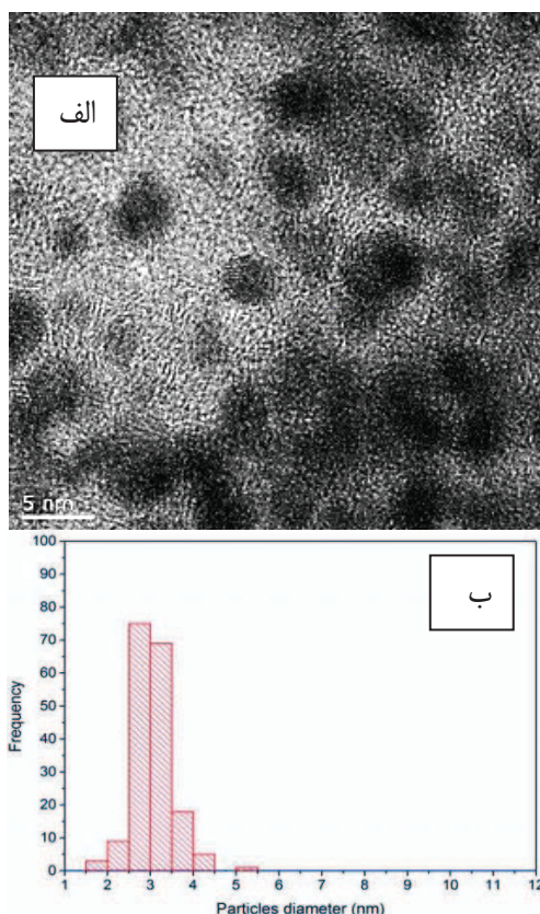
شکل ۲- الف) تصویر TEM از Au_{101}/AC فعال شده (شسته شده با تولوئن و پس از آن برشته شده در هوای ساکن در دمای ۱۰۰ درجه سانتی گراد به مدت ۳ ساعت) می باشد. ب) هیستوگرام توزیع اندازه ذرات است که اندازه متوسط ذرات طلا برابر 3 \pm 0.1 نانومتر تعیین شده است.
