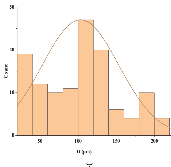
شکل ۵- منحنی توزیع اندازه تخلخل نمونه الف) ۱/۵-۴۰C-۱-۸۰۰ ب) ۳-۴۰C-۱-۸۰۰
