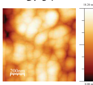
کاشت شده با جریان یونی 1 \times 10^{17}
