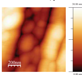
تانتالوم کاشت نشده
