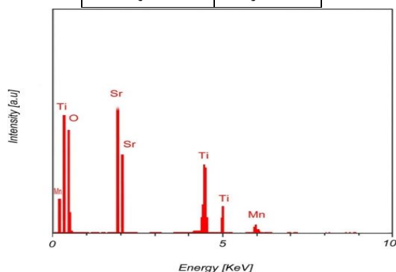
شکل ۳- تصویر طیفسنجی پراش پرتو الکترون کامپوزیت پروسکایت استرانسیوم تیتانات-منگنز
