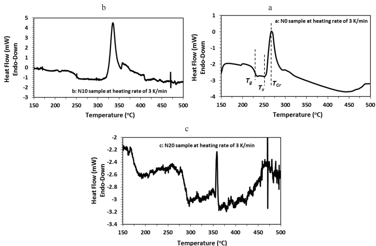
شکل ۲- ترموگراف‌های DSC برای نمونه‌های Nx در نرخ گرمایش ۳K/min؛
