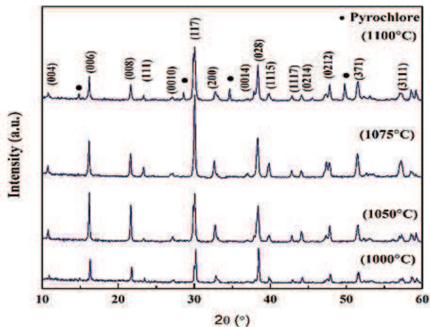
شکل ۲- الگوهای XRD مربوط به نمونه های تف جوشی شده در دماهای متفاوت.
